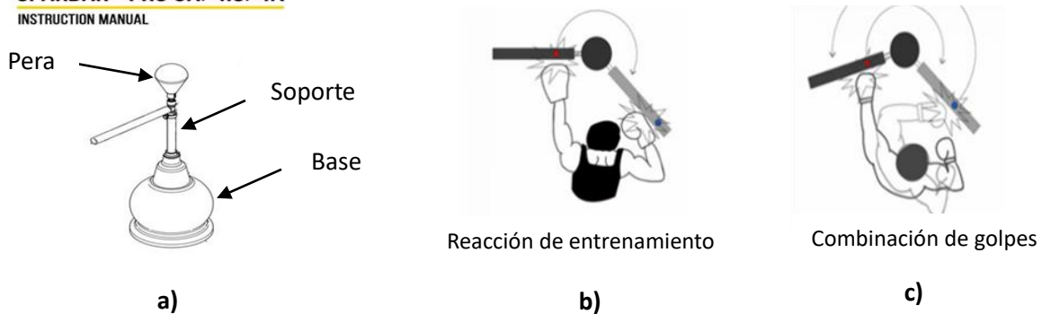
Figura 1.- Dispositivo SparBar Pro3X: a) Partes del dispositivo. b) Accionamiento del dispositivo (Postura de golpeo recto). c) Reacción del boxeador (postura de golpeo gancho).
