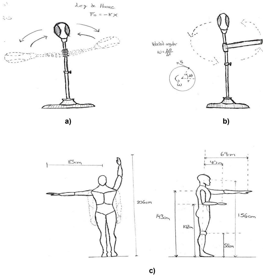
Figura 2.- Sistema de construcción del dispositivo (propia) a) Eje secundario con resorte y pera. b) Eje secundario con brazo de giro. c) Esquema antropométrico del boxeador mexicano promedio.
