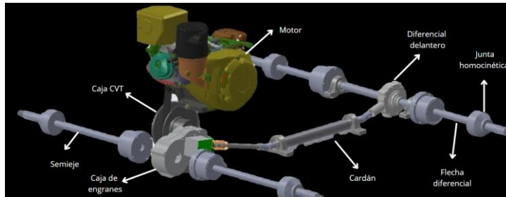
Figura 1. Tren de potencia [2].
