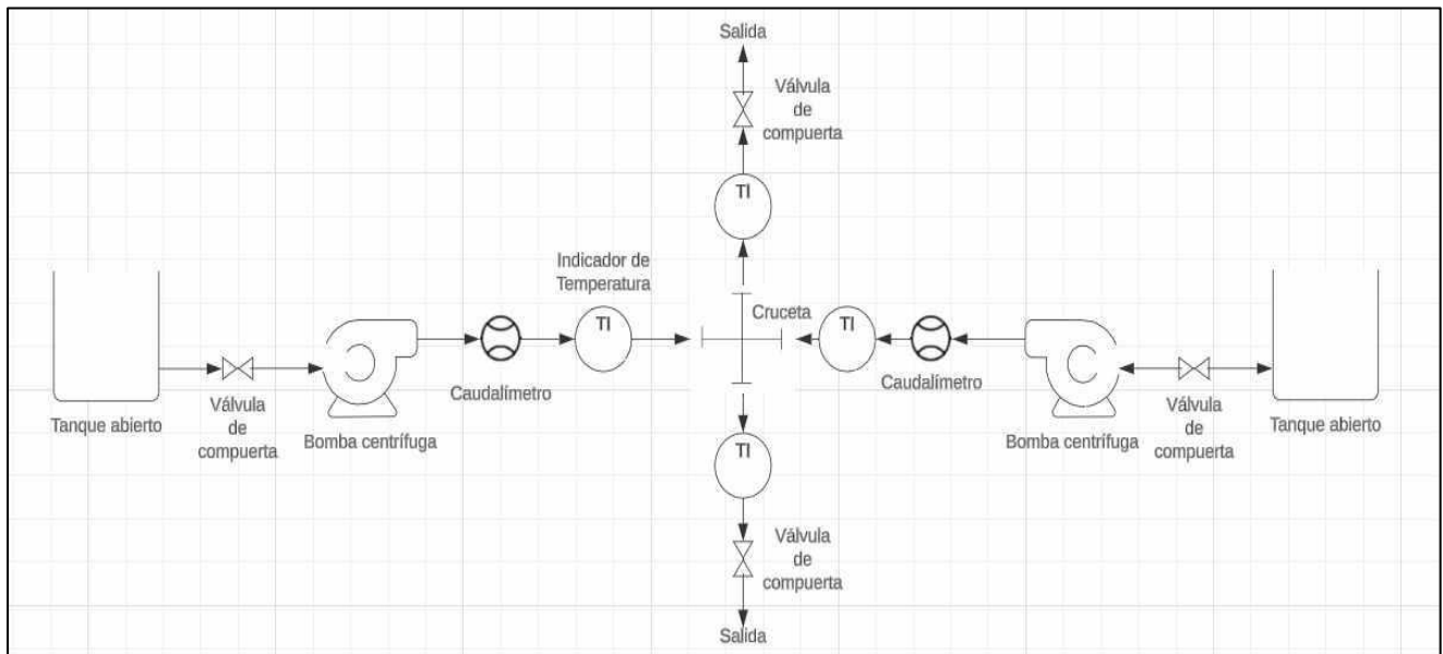
Figura 3. Diagrama de tubería e instrumentación simplificada.
